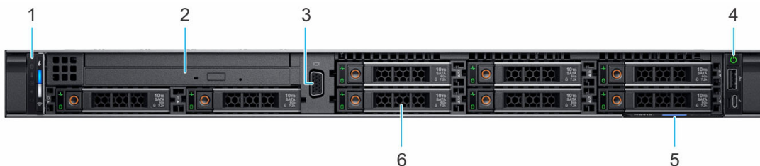
그림 2. 8개의 2.5" 드라이브 시스템의 전면
